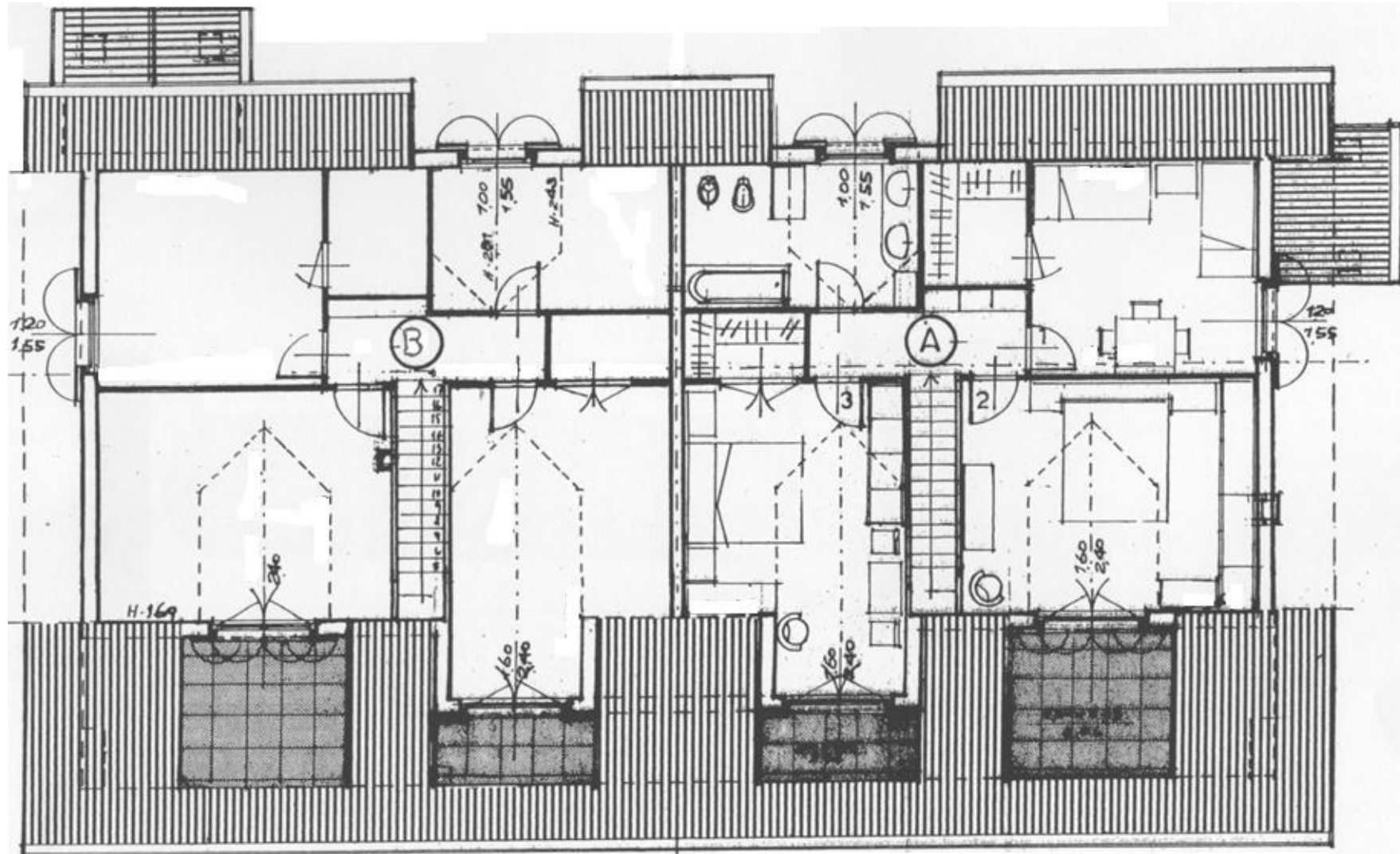
PIANO SOTTOTETTO ABITABILE
