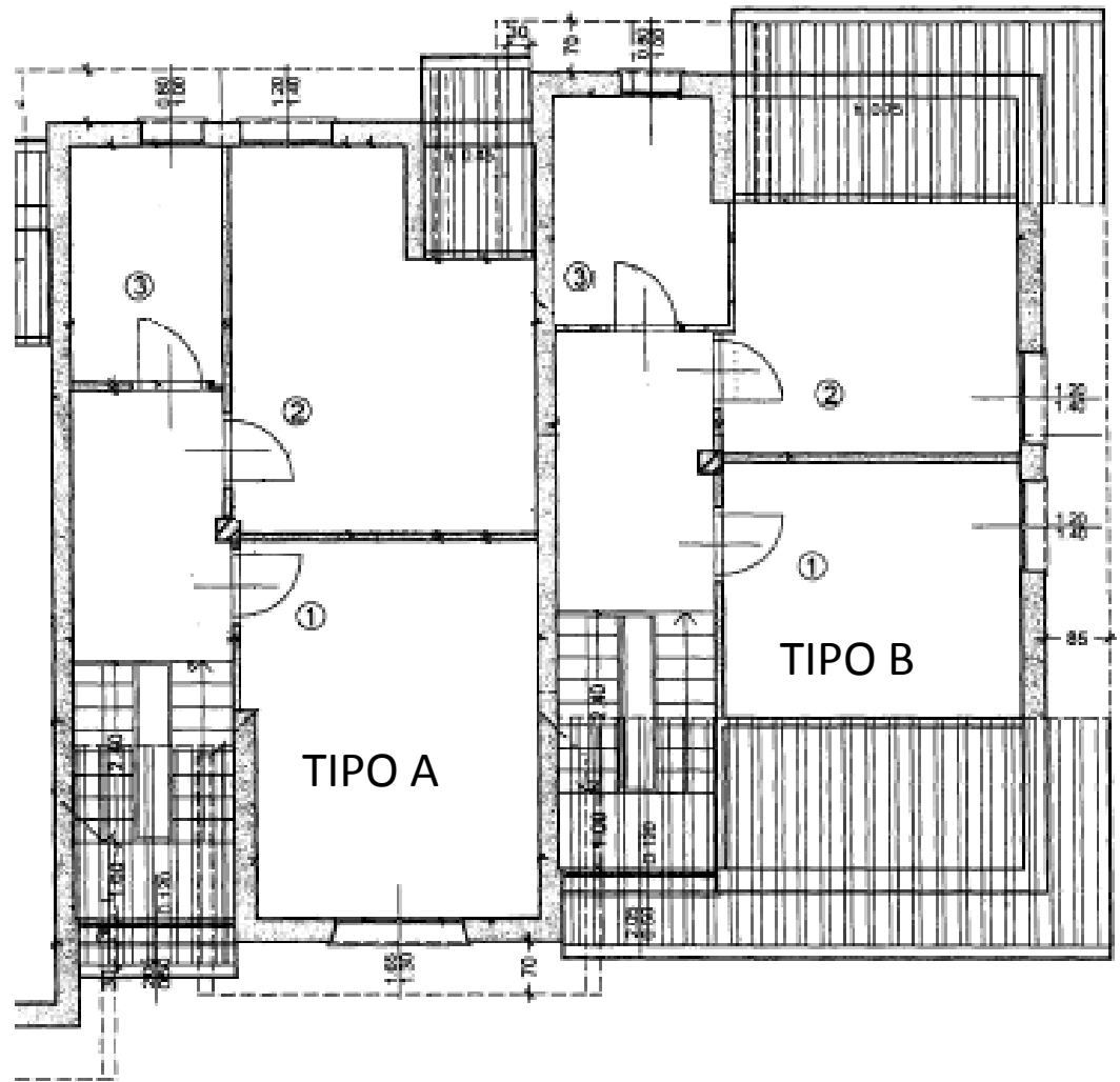
PIANO SOTTOTETTO
